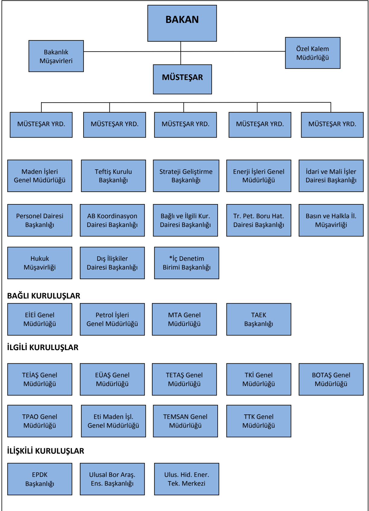
Şekil 1: Organizasyon Şeması
