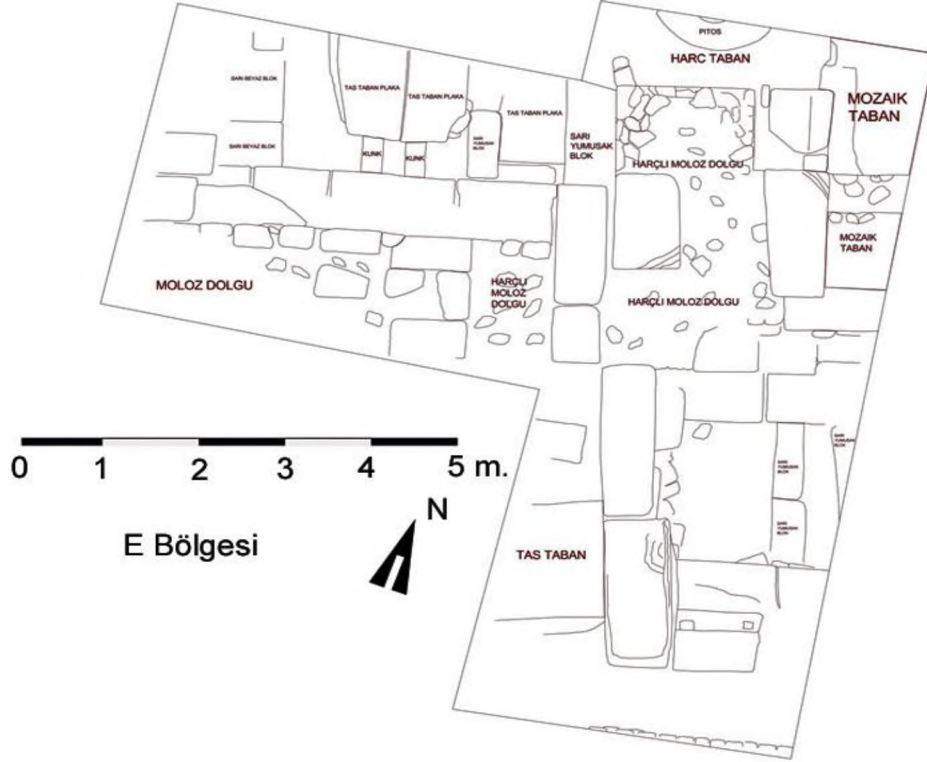
E Bölgesi 2013 çalışmaları neticesinde şekillenen taşplan rölovesi
